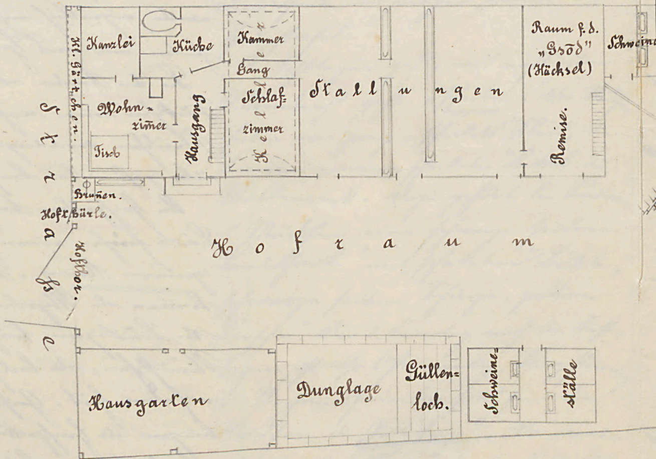
Erdgeschossgrundriß u. Situations-
